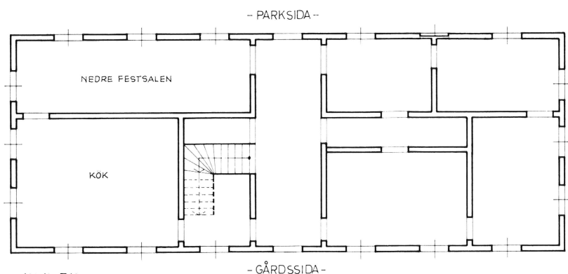
PLAN AV B.V.
