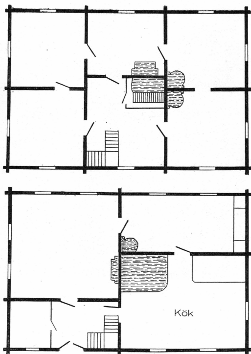
Bild 2. Manbyggnad i två våningar (bottenvåningen nedtill) på Siléns gård i Röcklinge. I köket skafferi på jällsängens plats, i sidkammaren sängalkov.
