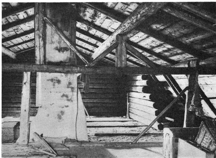
Bild 5. För att stödja de stora gavelröstena timras särskilda strävväggar på vinden. Gårdsjö n:o 1:3.
