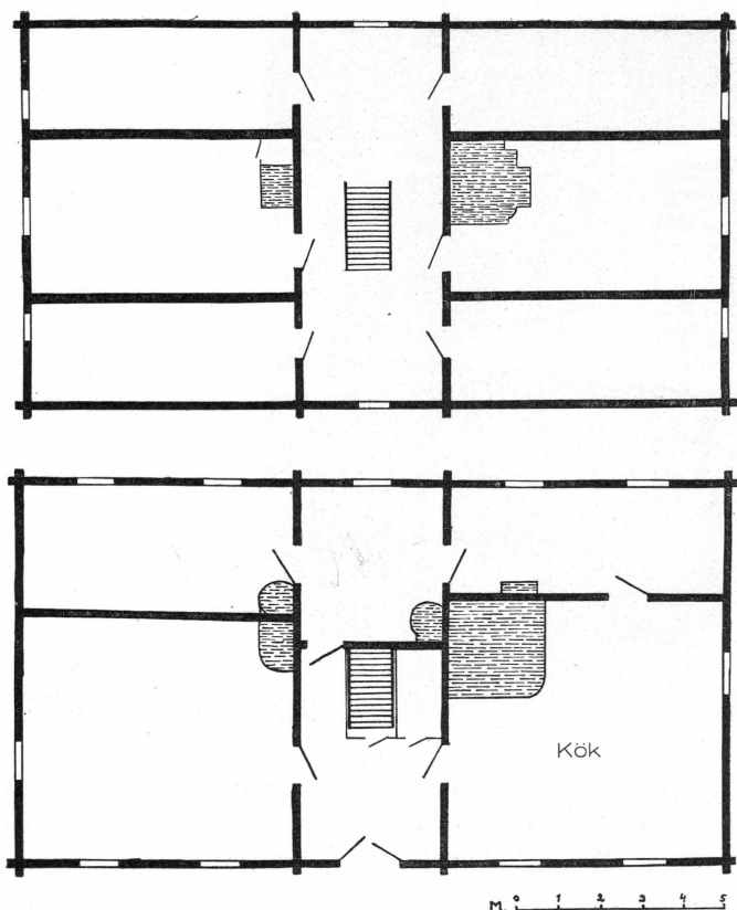
Bild 6. Manbyggnad på Sör Starfors n:o 2: 30. Nedtill bottenvåningen, däröver vindsvåningen.
