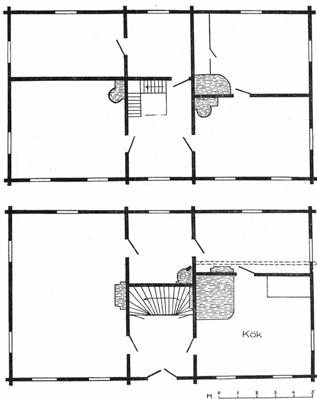
Bild 9. Manbyggnad i två våningar på Arnebo n:o 1 (bottenvåningen nedtill). Den prickade väggen anger sidkammareväggens ursprungliga läge. I köket jällsäng.
